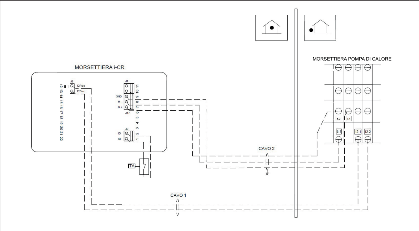
Esempio collegamento i-CR alla pompa di calore
